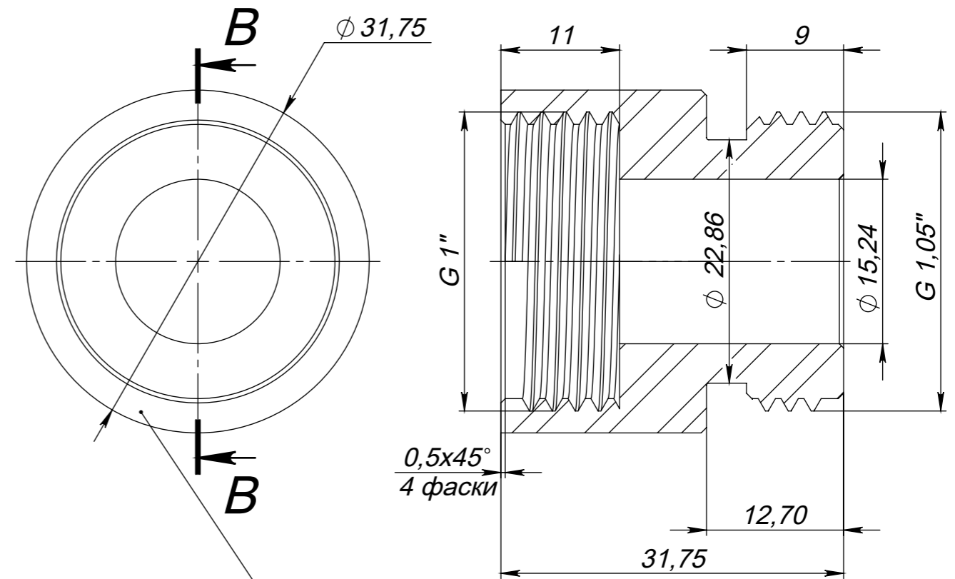
Переходник SM01 Материал: Латунь
