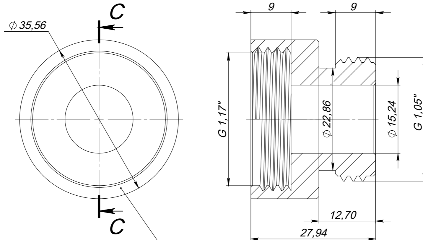
Переходник SM-XL Материал: Латунь
