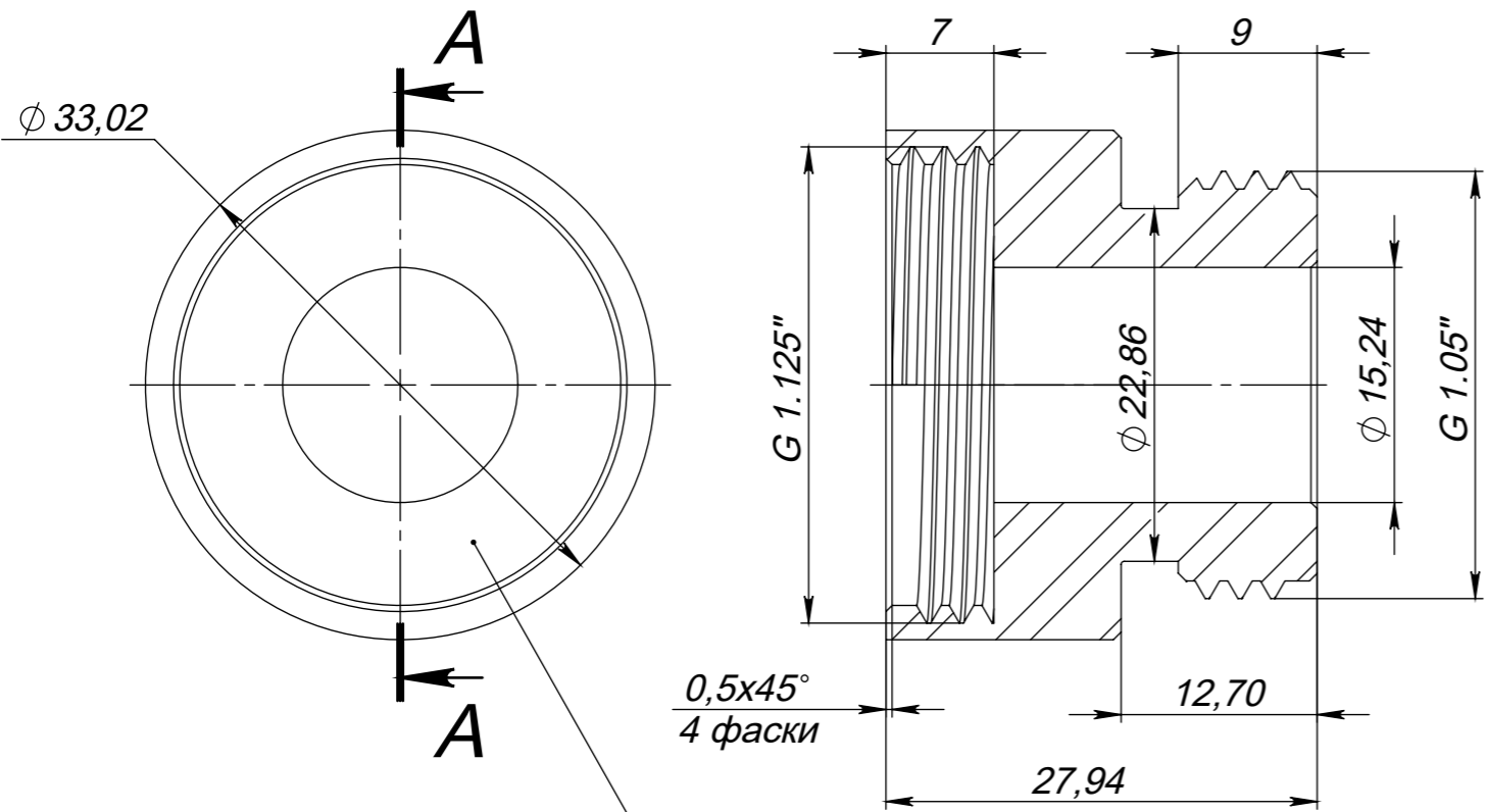
Переходник SM01.125 Материал: Латунь
